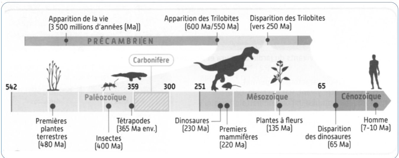
Document 3 : Frise simplifiée des temps géologiques
