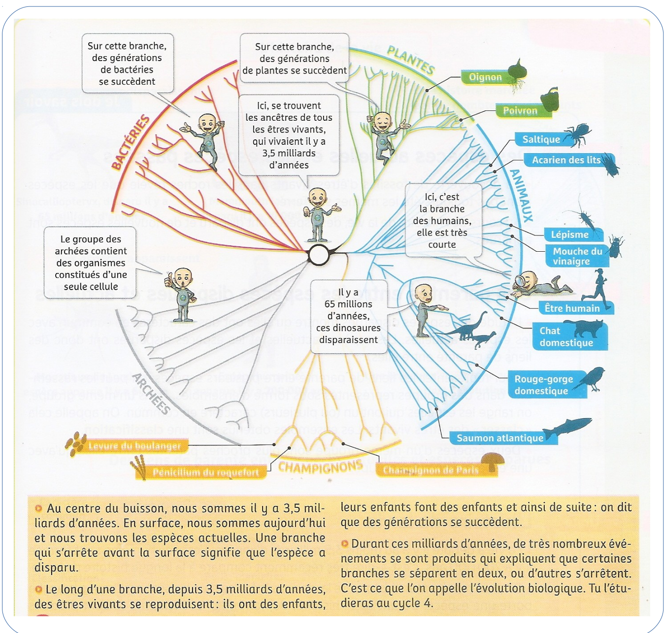
Document 4 : Schéma des liens de parenté entre les êtres vivants
