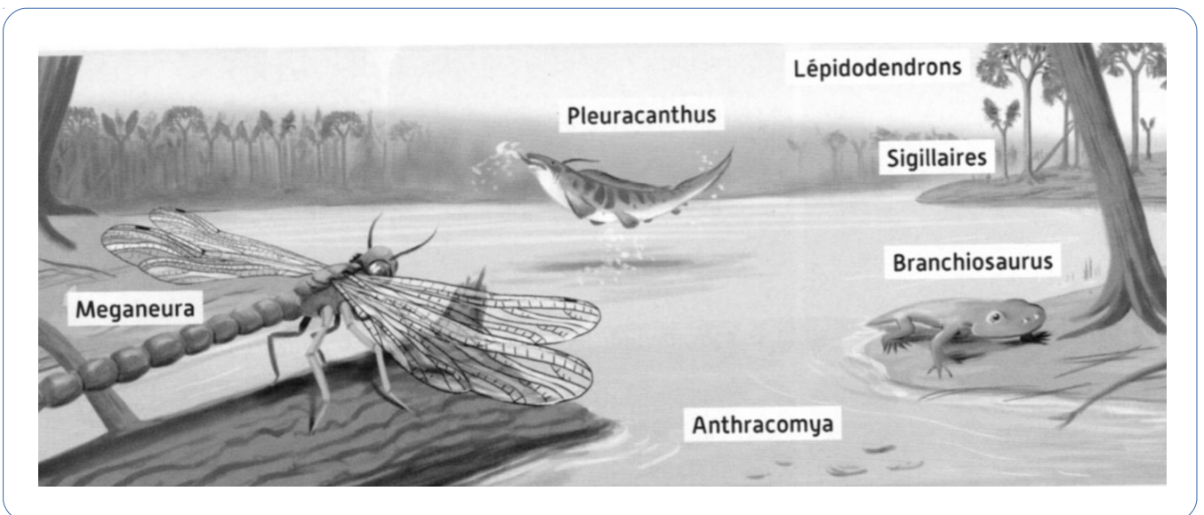
Document 2 Reconstitution d'un paysage marécageux ancien d'il y a 300 millions d'années
