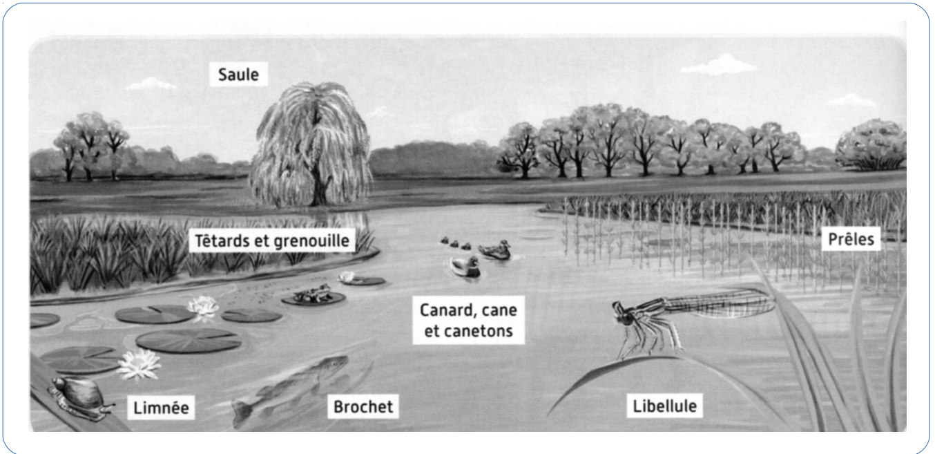
Document 1 Paysage marécageux actuel
