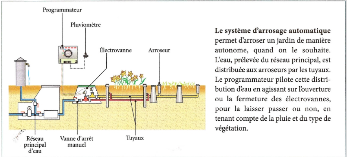
DOC. 1 Principe du système d'arrosage automatique de jardin
